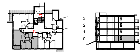
ZESTAWIENIE POMIESZCZEŃ
